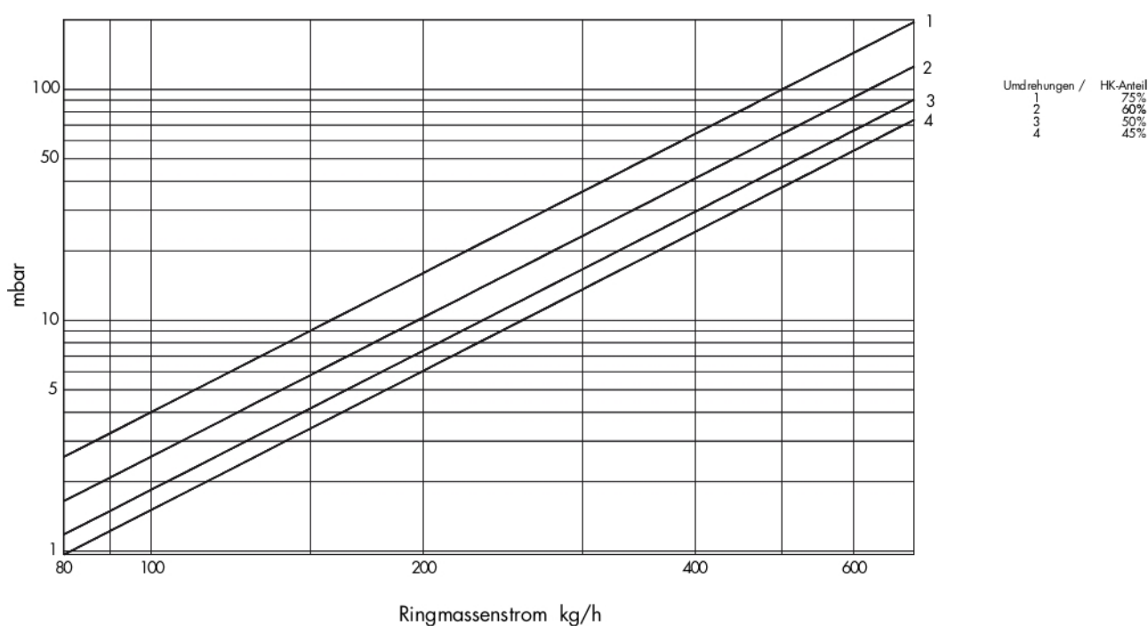
Einrohrumlenkstück Eckform absperrrbar Artikel-Nr. 2257002601 / 2257002701
